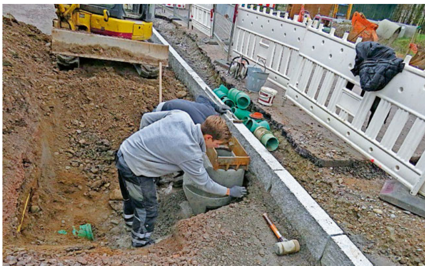
Ein Straßeneinlauf wird gesetzt
