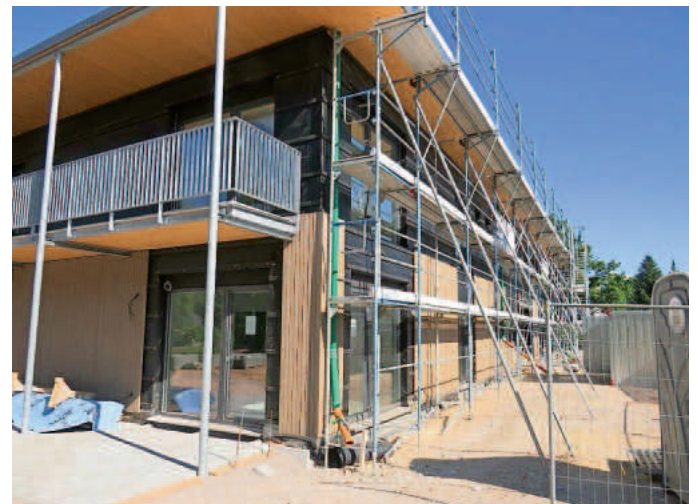
Die Fertigstellung der Holzschalung an der Fassade
